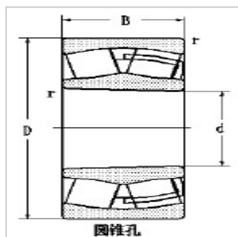
圆锥孔
